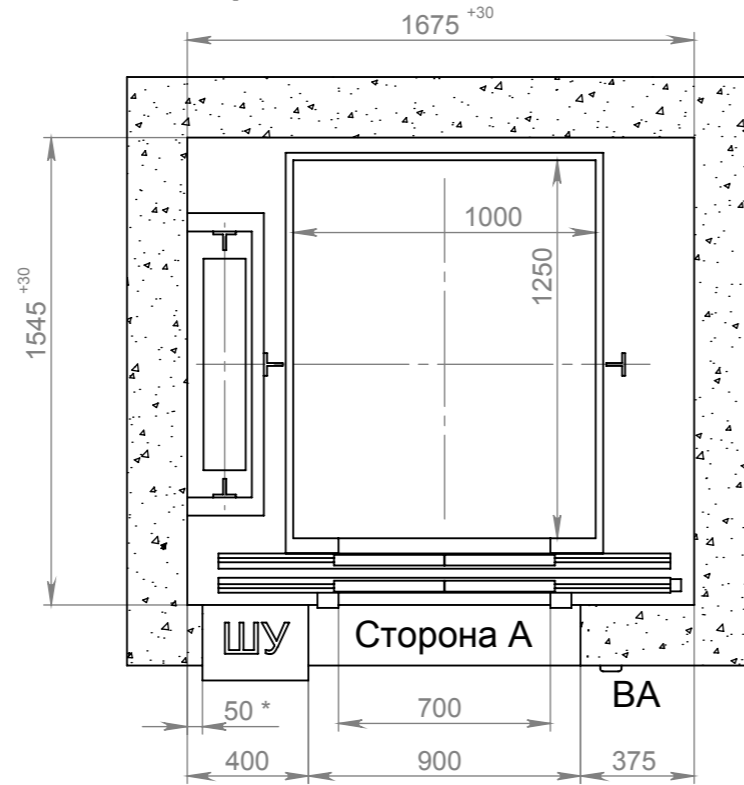
UW 450R-1.0(1.6)-CO 070 Противовес слева
