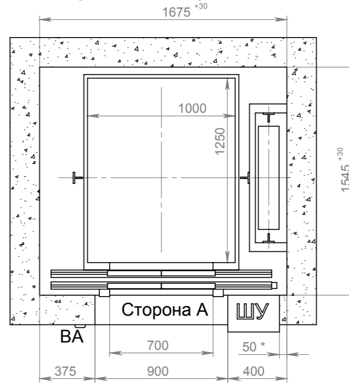
UW 450R-1.0(1.6)-CO 070 Противовес справа
