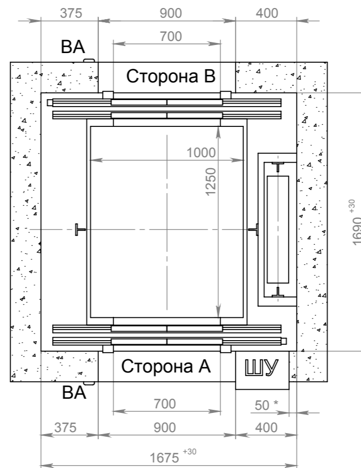
UW 450R-1.0(1.6)-2CO 070 Противовес справа
